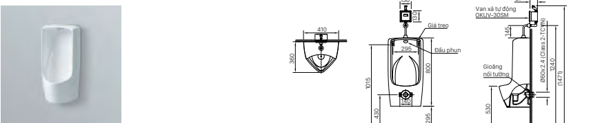
AU-411V | U-411V (VAN XẢ TỰ ĐỘNG OKUV-30SM)
