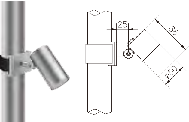
SL1146H 适配树杆尺寸(60-200)MM
