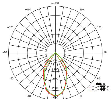
平均光束角(50%): 63.9° 01.150.00
