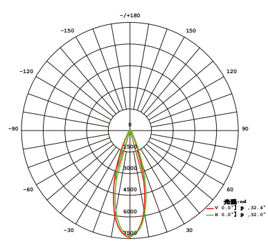
平均光束角 (50%) : 32.2 度 SL1140 30°
