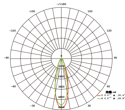
平均光束角 (50%) : 29.6 度 SL1136 30°
