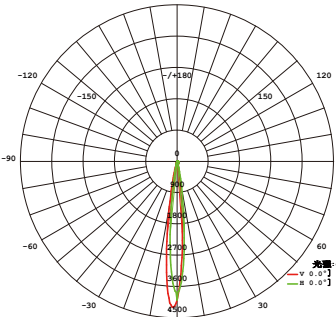
平均光通量 (50%) : 12.4° SL1105 12.5°
