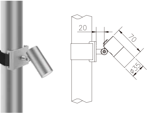
SL1147H 适配树杆尺寸(60–200)MM
