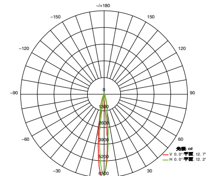
平均光束角(50%): 12.4° SL1139 12.5°
