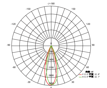
平均光束角(50%): 32.5° SL1139 30°
