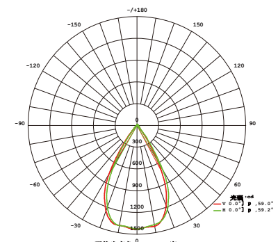
平均光束角 (50%) : 59.1 度 SL1140 60°
