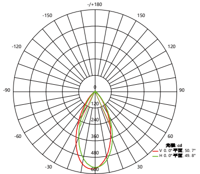
平均光束角(50%): 50.2 度 SL1145 60°
