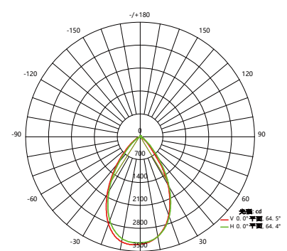
平均光束角 (50%) : 64.5 度 SL1136 60°
