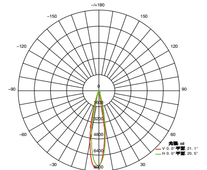
平均光束角(50%): 20.8° SL1139 20°
