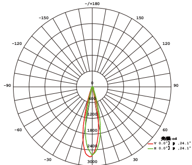
平均光束角(50%): 24.1 度 SL1145 24°
