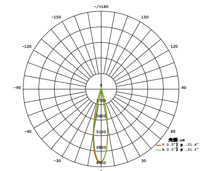
平均光束角(50%): 21.4° SL1139 22.5°
