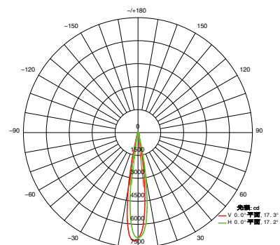
平均光束角 (50%) : 17.2 度 SL1140 20°
