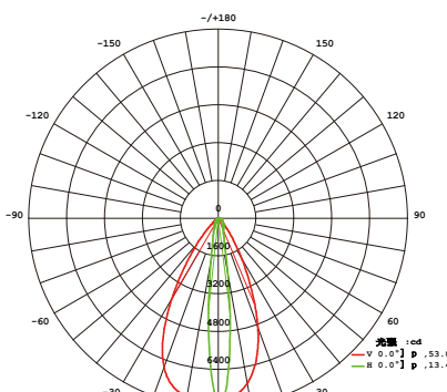
平均光束角 (50%) : 33.2° SL1136 10x70°
