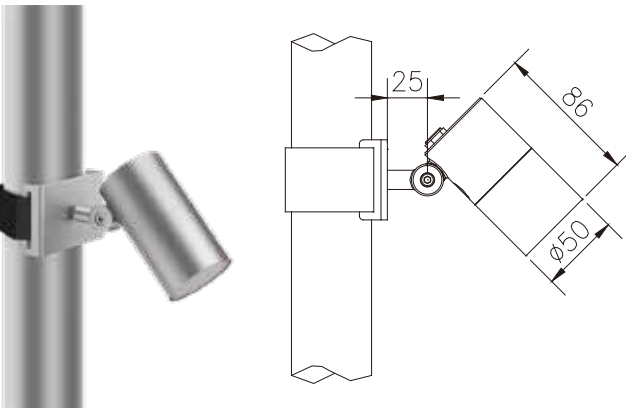
SL1146H 适配树杆尺寸(60-200)MM
