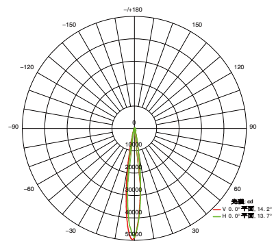
平均光束角 (50%) : 13.9 度 SL1136 12°
