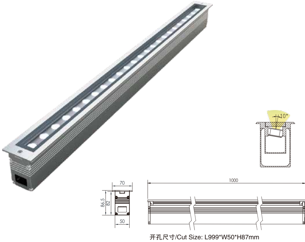
开孔尺寸/Cut Size: L999*W50*H87mm
