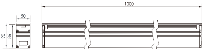
开孔尺寸/Cut Size: L999*W50*H87mm
