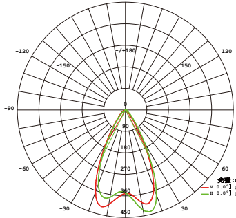
平均光通量 (50%) : 57.8° SL1105 60°
