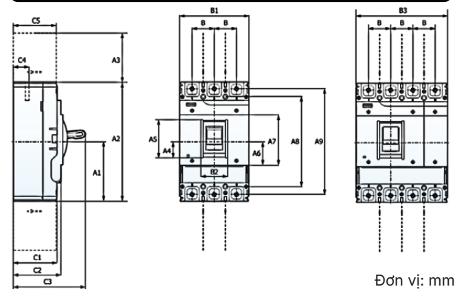
Kích thước MCCB SF Series
