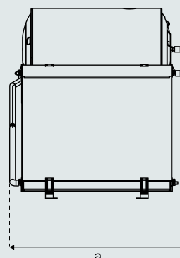
MẶT TRƯỚC
