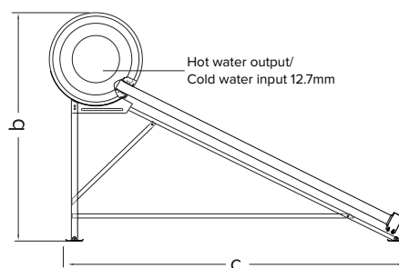
MẶT BÊN
