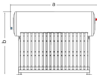
MẶT TRƯỚC
